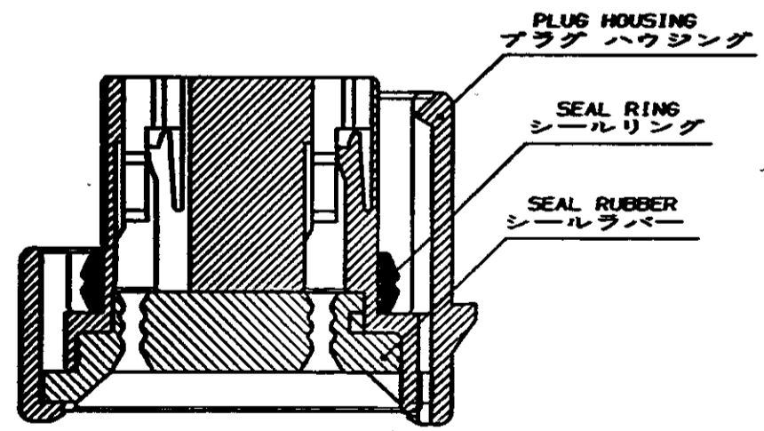
SECTION 断面 A-A SCALE: 2/1
